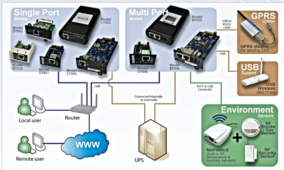
NetAgent9: Web interface
